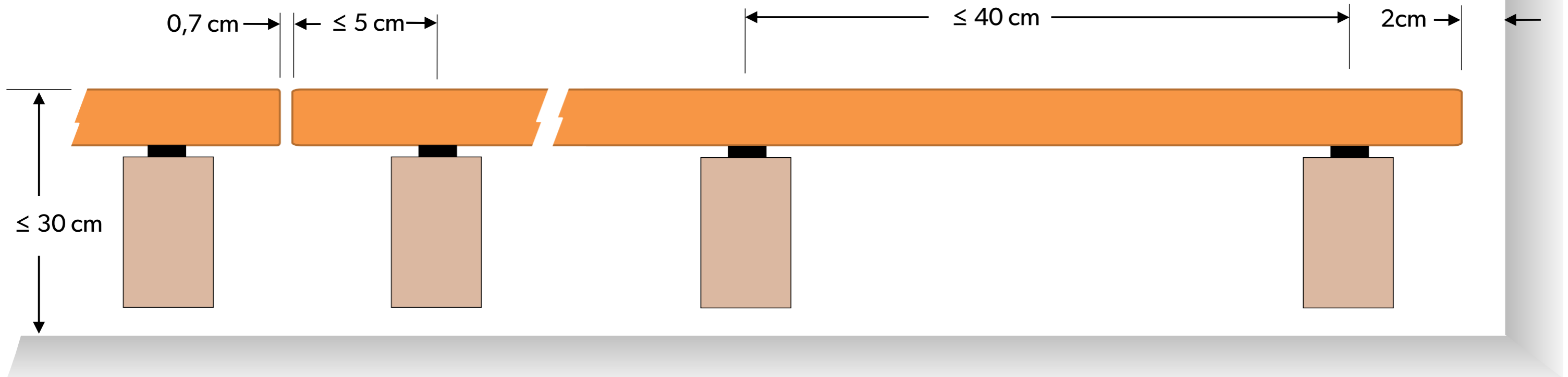
Verlegemaße:
